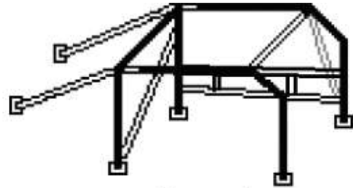
Alternative 2 Beidseitig A-Säule zu B-Säule und B-Säule zu B-Säule
